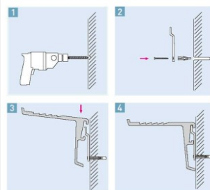
Einfache Wandbefestigung inkl. Montagematerial
